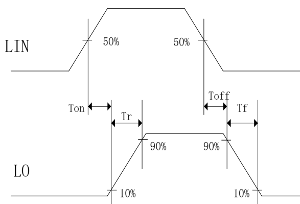
图 7-1. 输出 L0 开关时间波形图
