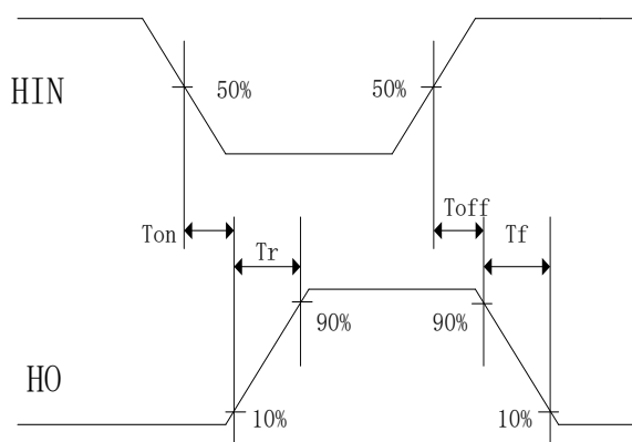
7-2. 输出 H0 开关时间波形图
